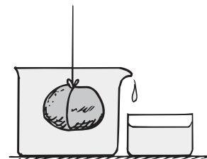
FIGURA 13.10 Cuando se sumerge una piedra, desplaza agua cuyo volumen es igual al volumen de la piedra.
