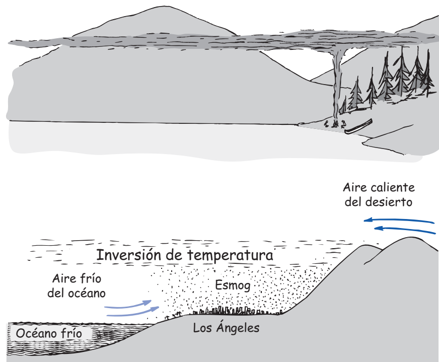
FIGURA 18.9 El esmog de Los Ángeles queda atrapado por las montañas y por una inversión térmica causada por el aire cálido del desierto de Mojave, que está arriba del aire frío del Océano Pacífico.
