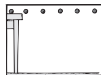
Movimiento horizontal sin gravedad
