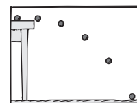
Movimientos horizontal y vertical combinados
