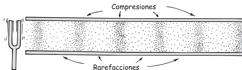
FIGURA 20.2 Las compresiones y las rarefacciones se propagan (a la misma rapidez y en la misma dirección) desde el diapasón, por el aire en el tubo.
