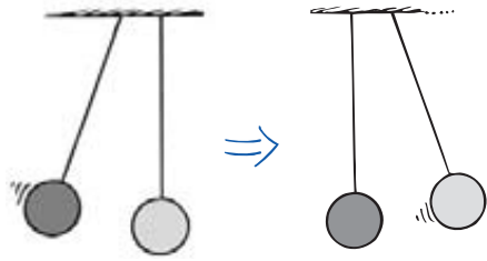
FIGURA 5.5 Las fuerzas de impacto entre las esferas de la izquierda y de la derecha mueven una y detienen la otra.
