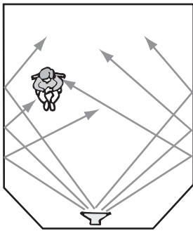
FIGURA 20.6 El ángulo del sonido incidente es igual al ángulo del sonido reflejado.
