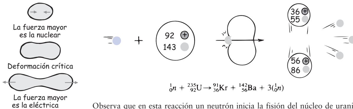
FIGURA 34.1 La deformación nuclear puede dar como resultado que las fuerzas eléctricas de repulsión superen la fuerza nuclear de atracción, en cuyo caso se produce la fisión.
