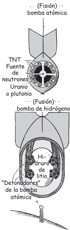
FIGURA 34.22 Bombas de fisión y de fusión.
