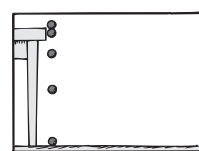
Movimiento vertical sólo con gravedad
