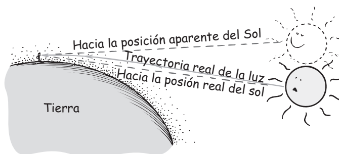
FIGURA 28.19 Debido a la refracción atmosférica, cuando el Sol está cerca del horizonte, parece que está más alto en el cielo.
