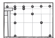
Superposición de los casos precedentes
