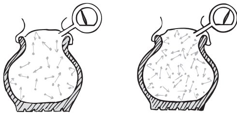
FIGURA 14.12 Cuando aumenta la densidad del aire en el neumático, aumenta su presión.
