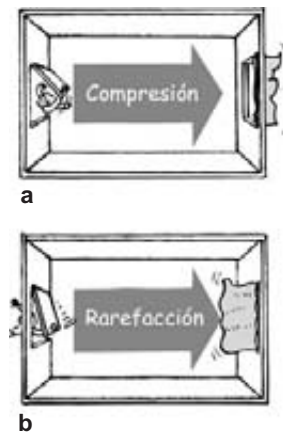
FIGURA 20.1 a) Cuando la puerta se abre, se produce una compresión que se propaga por el recinto. b) Cuando la puerta se cierra, se produce un rarefacción o enrarecimiento que se propaga por el recinto. (Adaptada de A. V. Baez, The New College Physics: A Spiral Approach . San Francisco: W. H. Freeman and Company. Copyright © 1967.)
